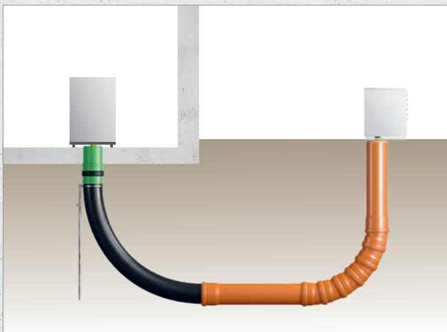
Systematische Darstellung: Einbau Quadro-Sicura® E-BP/SRB
