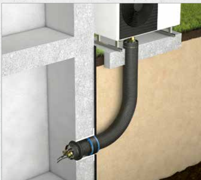
Systematische Darstellung: Einbau DOYMAfix® Connect HP/B
