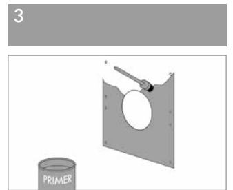
Grundierung Sika Primer-3N im Bereich des Futterrohres mit Hilfe eines Pinsels auf die Wand auftragen.
