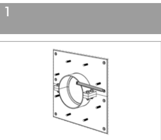
Geteiltes Futterrohr zusammenmontiert an der Wand positionieren und Dübellöcher anzeichnen.
