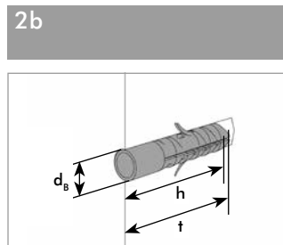
Mindest-Bohrlochtiefe t \geq 70 mm Dübellänge h = 50 mm Bohr-/Lochdurchmesser d_B = 10 mm
