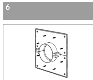
Futterrohr an der Wand montieren, Schrauben setzen und anziehen. Hinweis: Zur Kontrolle der richtigen Montage sollte beim Anziehen der Schrauben umlaufend innen und außen, sowie aus allen Bohrungen der Platte Dichtmasse herausquellen.
