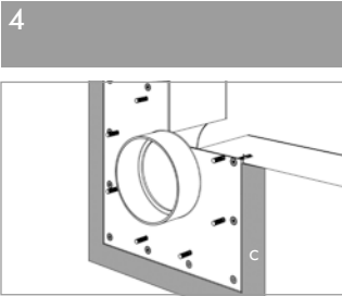
Ausgleich des Überganges vom Festflansch zur Wand mit Mörtel (C).
