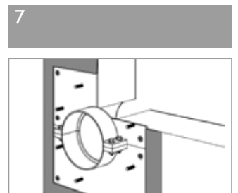
Ausgleich des Überganges vom Festflansch zur Wand mit Mörtel (C).
