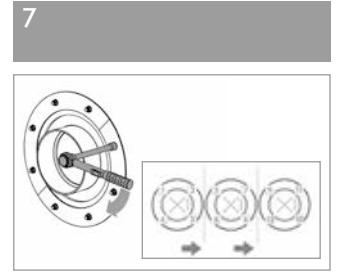
Muttern mehrfach über Kreuz anziehen. Drehmomente siehe Tabelle, Rückseite (Auszug aus DIN 18195/DIN 18533 bzw. nach Angaben der Bahnenhersteller).
