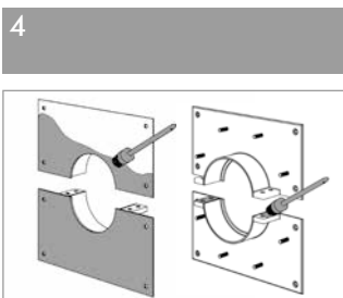
Sika Haftreiniger-1 auf die Rückseite des Festflansches (entgegen der Hülse) und auf die Teilungslaschen mit Hilfe eines Pinsels oder Tuches auftragen.
