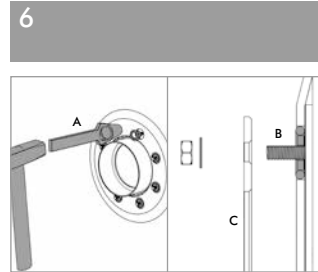
KMB nach dem Trocknen mittels Loch-eisen (A) zentrisch um die Bolzen herum ausstanzen (Ø 40 mm bei M12, Ø 55 mm bei M20). Distanzscheiben und O-Ringe (B) einlegen. Beide Hälften des Losflansches (C) mit der Fase bzw. besandeter Fläche in Richtung KMB aufsetzen, U-Scheiben und Muttern montieren.
